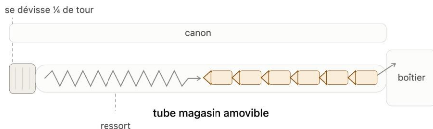
Schéma d'un tube magasin amovible sur une carabine à levier de sous-garde.
